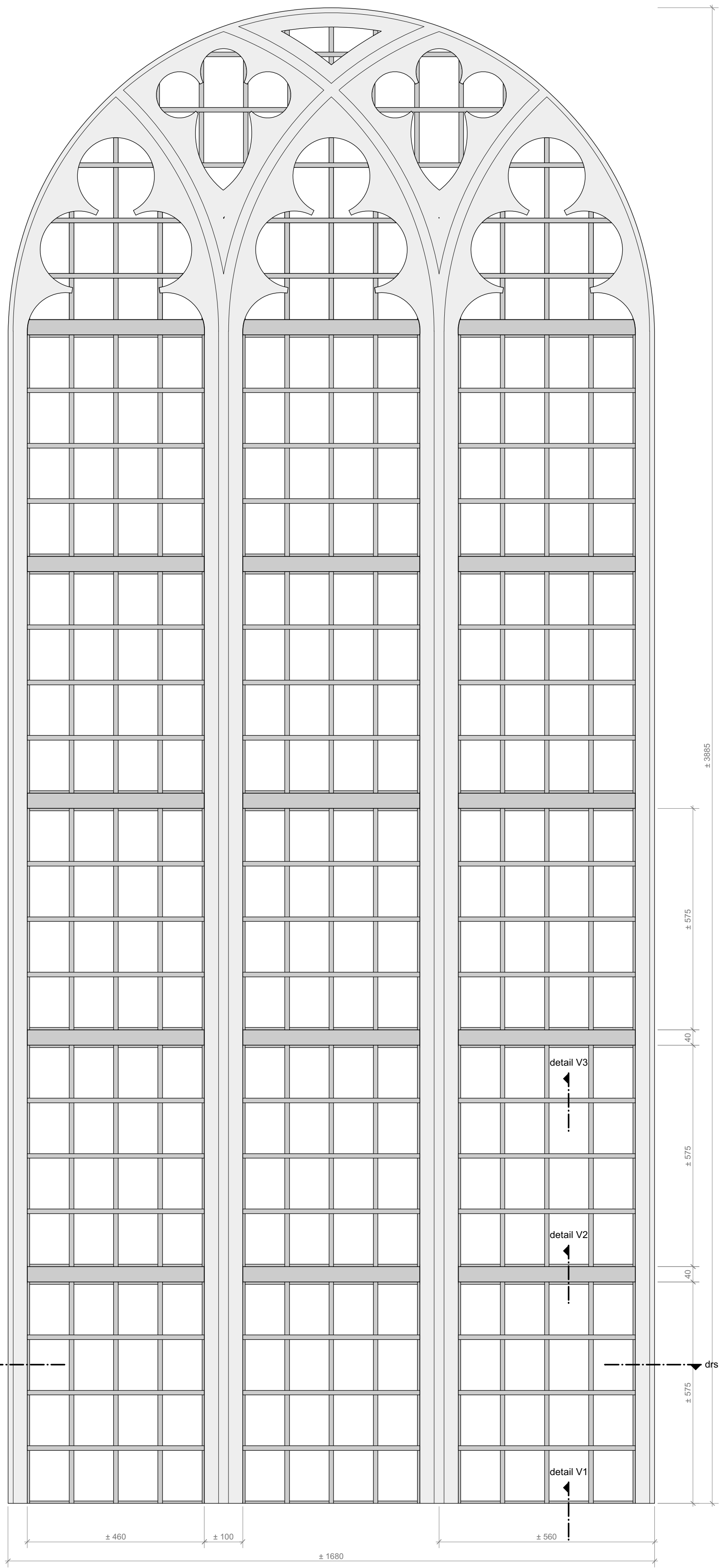
Aanzicht binnenzijde (blank glas) Venster Heilig Graf (schaal 1:8)
