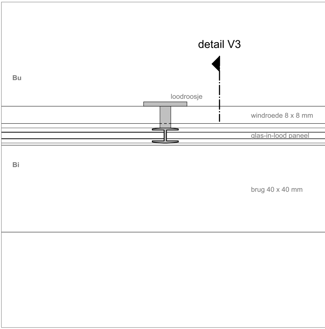
Bestaande situatie - Detail H1
