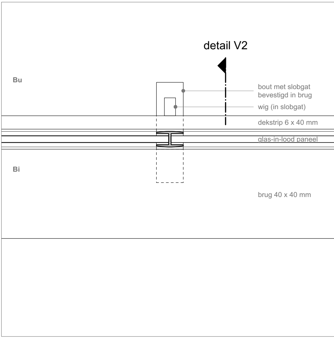
Bestaande situatie - Detail H2
