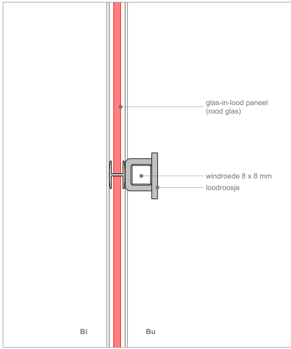
Expositie situatie - Detail V3
