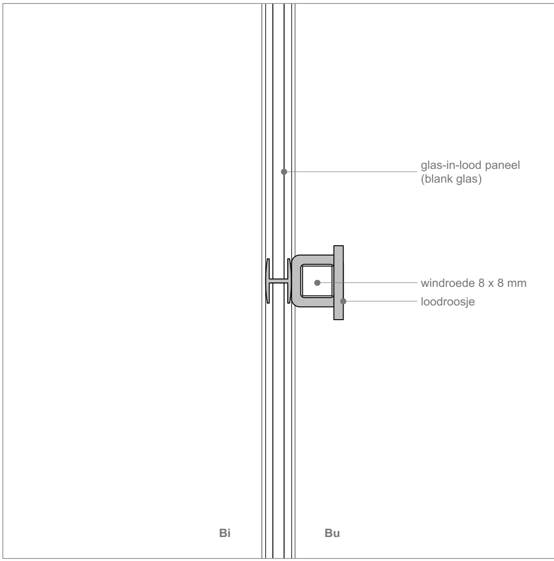
Bestaande situatie - Detail V3
