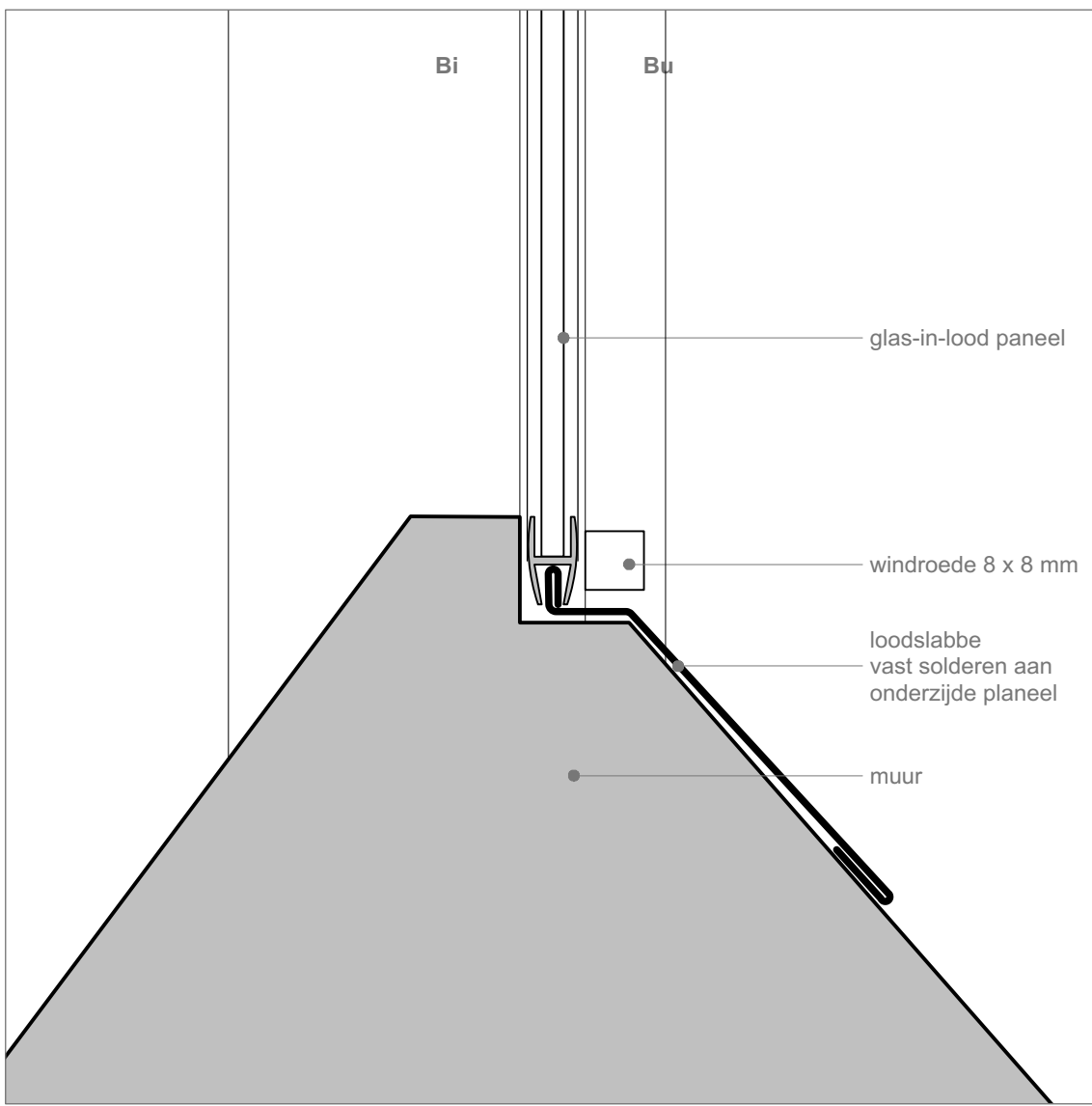
Bestaande situatie - Detail V1
