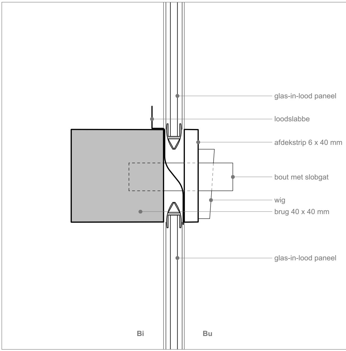
Bestaande situatie - Detail V2
